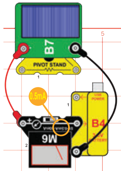
Regulacja kąta względem źródła światła i pomiar prądu ładowania:
